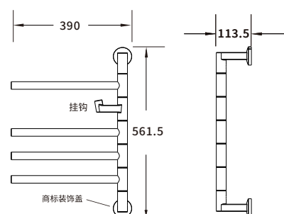
K-29349T/K-29349T-S/K-29349T-A/K-29349T-ZZ/K-29349T-ZA(带挂钩) P29349T/P29349T-A/P29349T-S(带挂钩) K-29355T/K-29355T-S/K-29355T-A(无挂钩) P29355T/P29355T-A/P29355T-S(无挂钩)
